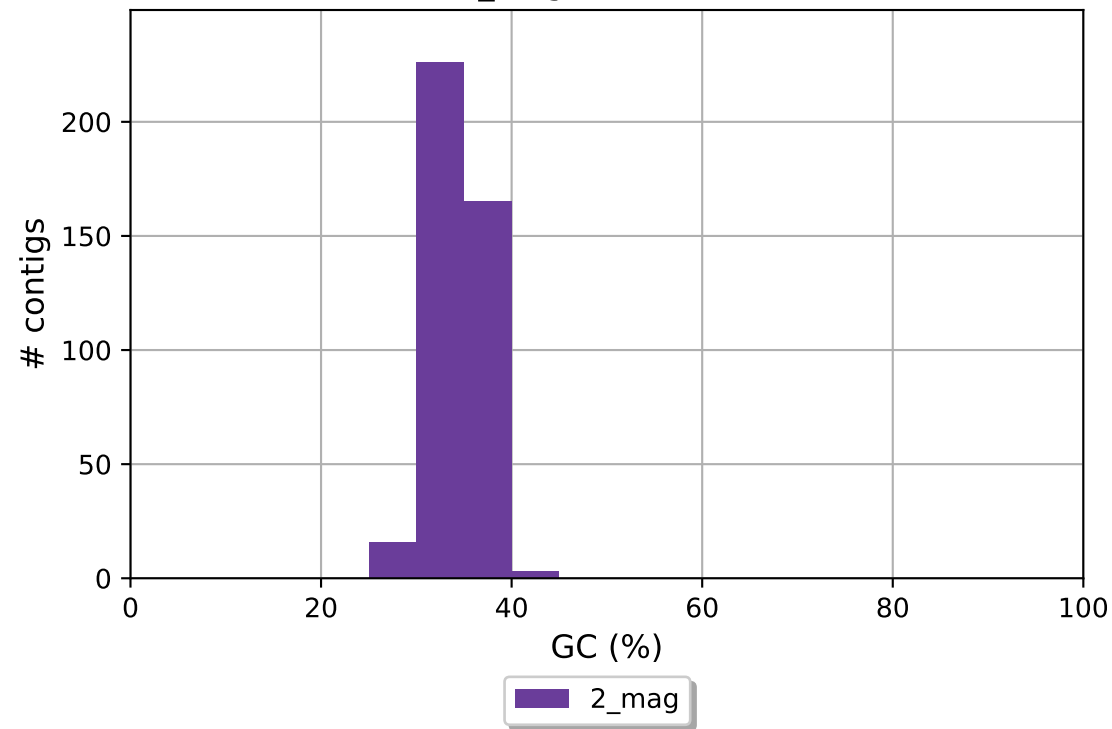
2_mag GC content
