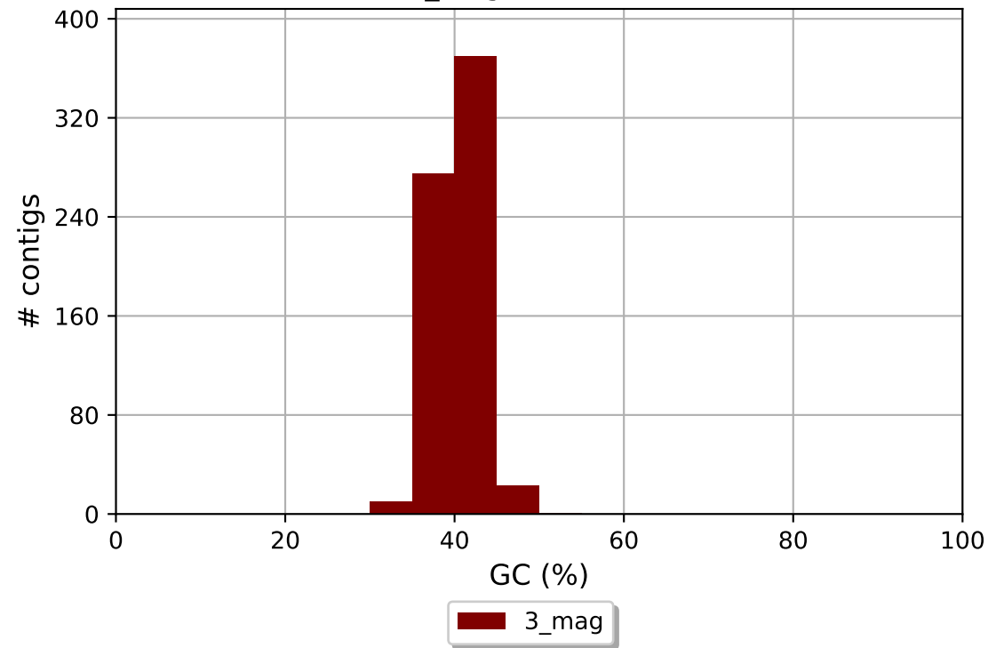
3_mag GC content
