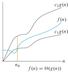
Figura 2: Cota Ajustada \Theta(g(n))
