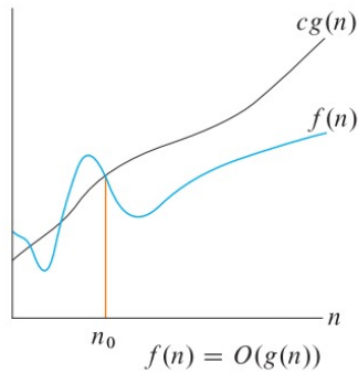
Figura 1: Cota Superior O(g(n))
