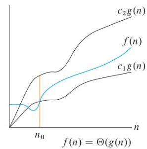
Figura 3: Análisis de \Theta(g(n))
