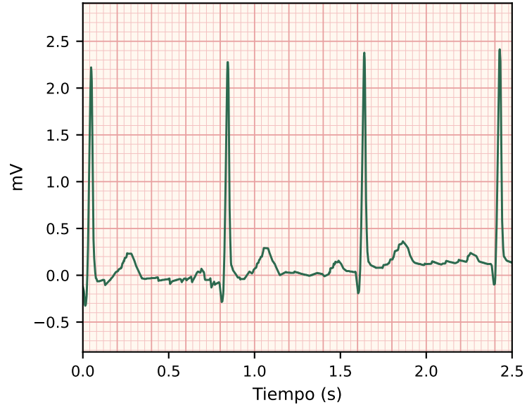
HYP
