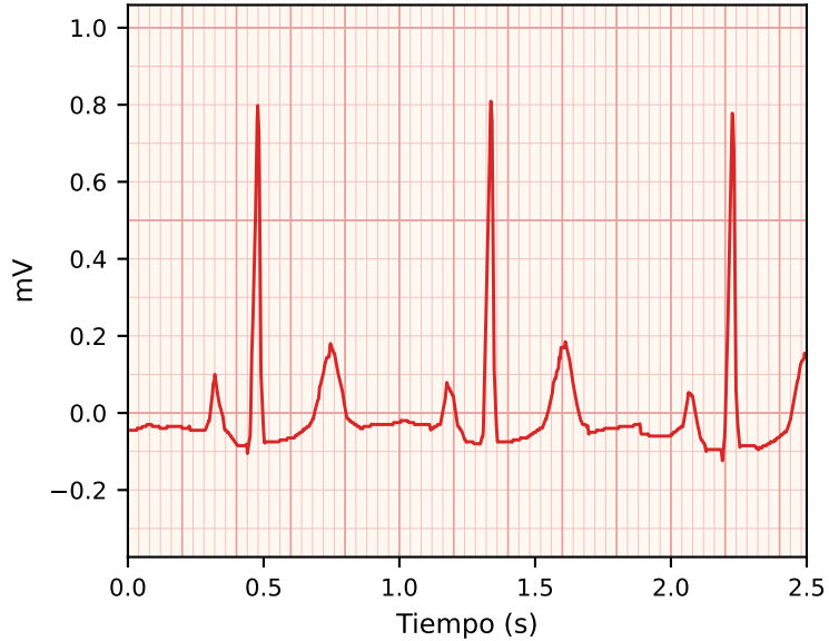
MI
