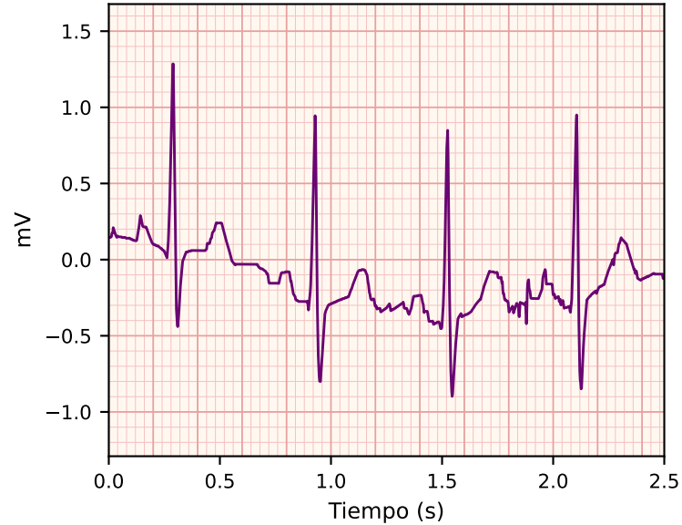
CD
