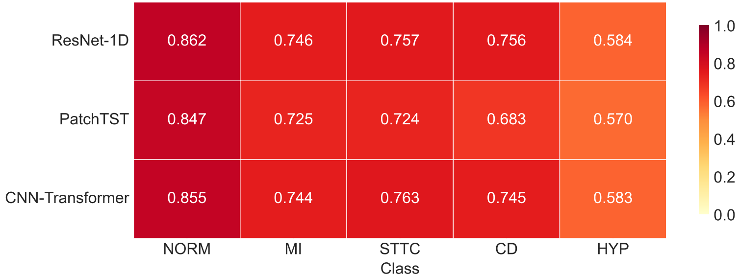
F1 Score per Class per Model
