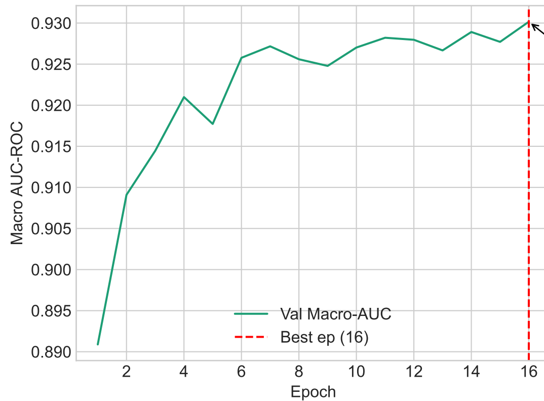
Validation Macro AUC
