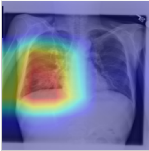
camada denseblock4
