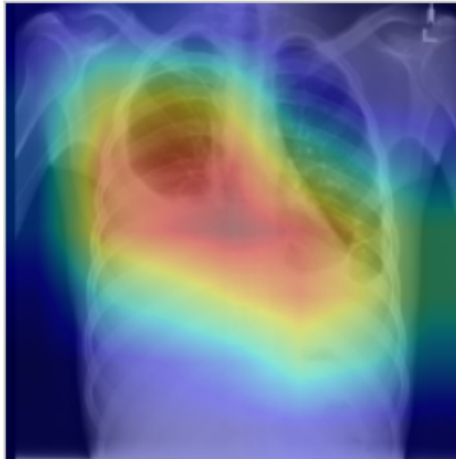
camada denseblock4
