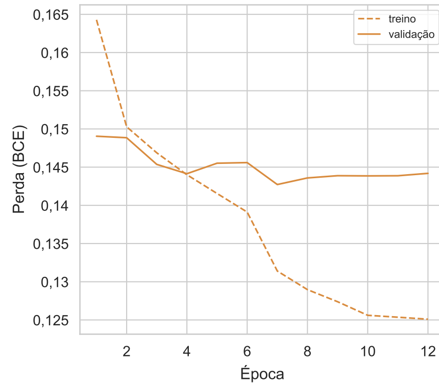
Perda: e1_baseline_seed43
