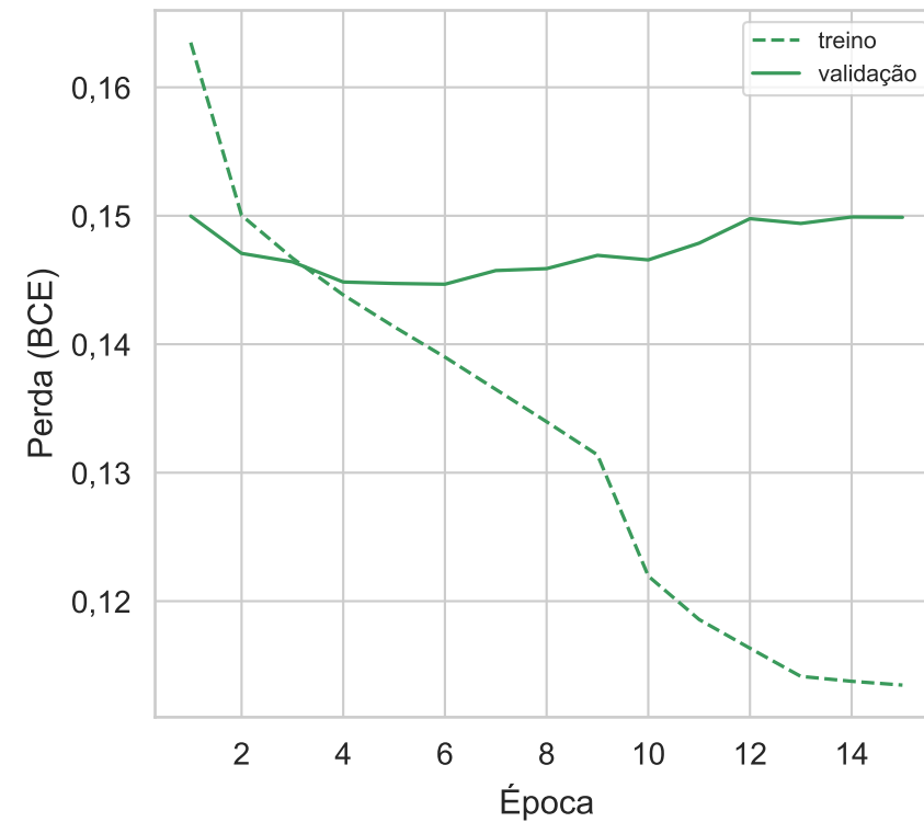
Perda: e1_baseline_seed44
