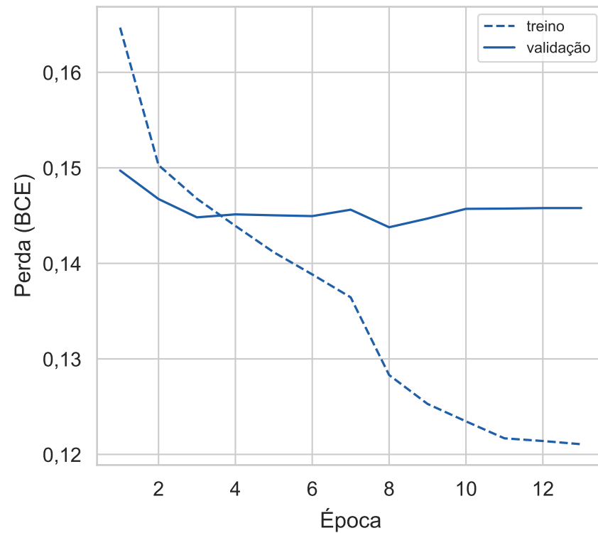
Perda: e1_baseline
