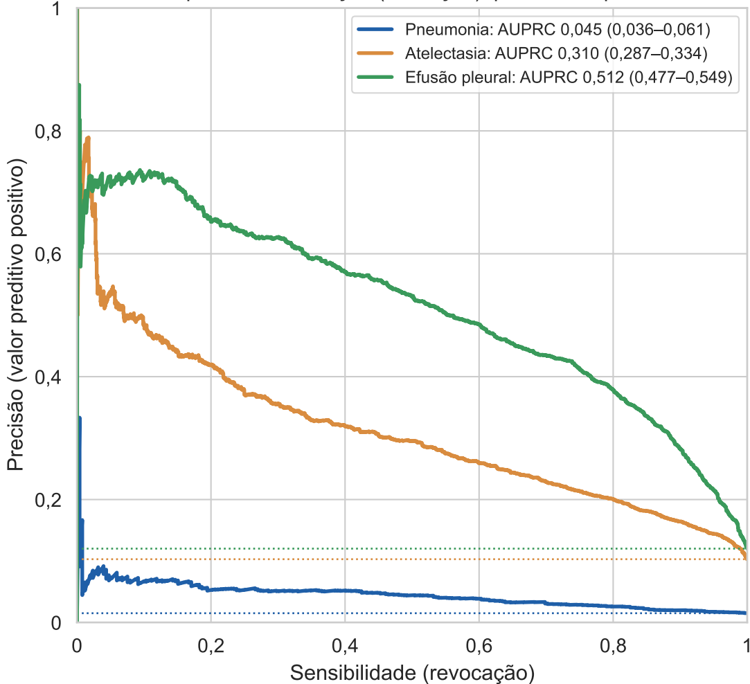
Curvas precisão-revocação (validação); pontilhado: prevalência
