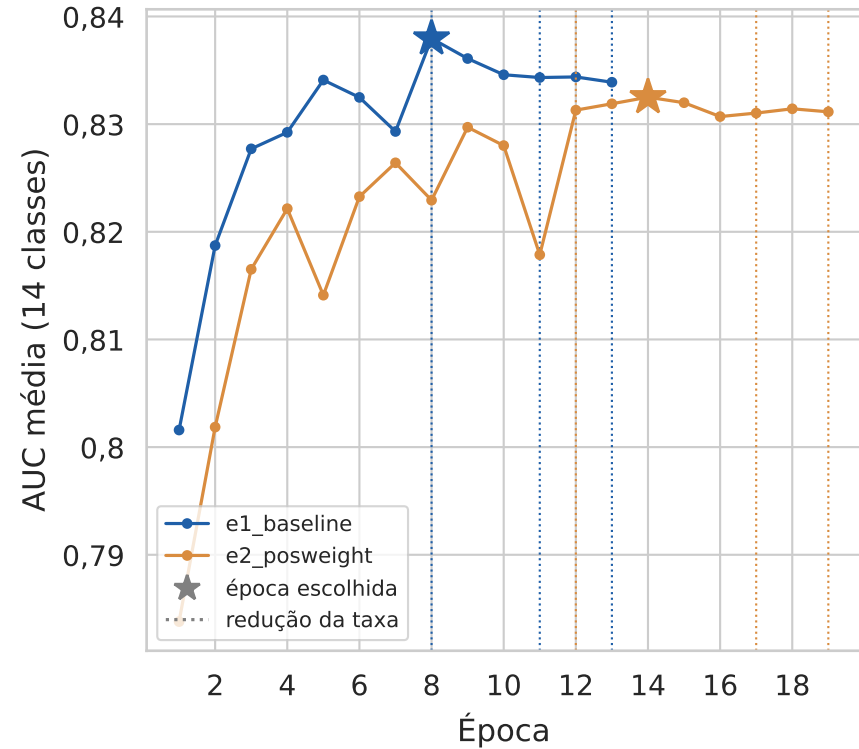
AUC média de validação
