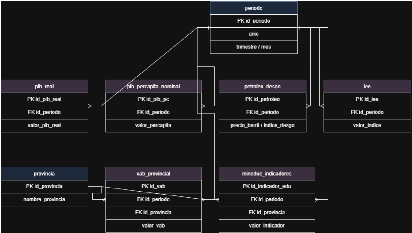
Figura 2. Modelo entidad-relación propuesto para la capa Silver.
