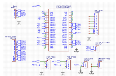
Figura 14: Esquemático.
