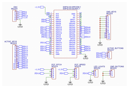
Figura 14: Esquemático.
