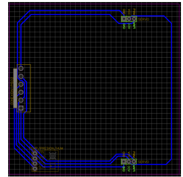
Figura 8: PCB del piso 3: BME280 y servos.
