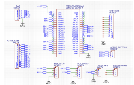
Figura 14: Esquemático de la PCB.
