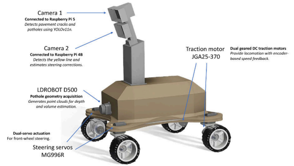
Figura 1: Modelo 3D del rover: Cámaras, LiDAR D500, motores de tracción y servos de dirección.
