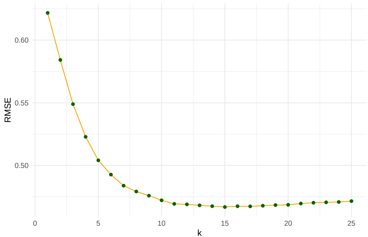
Valor de k vs. RMSE
