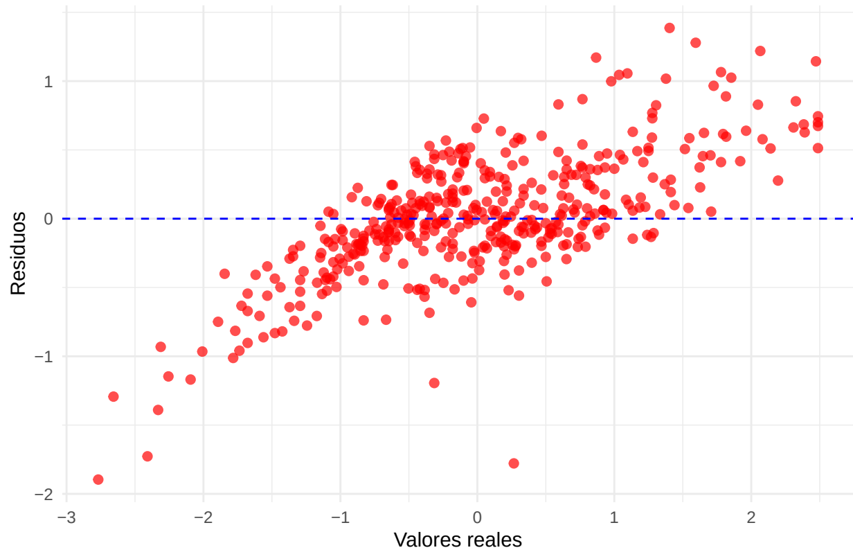
Residuos vs. Valores reales
