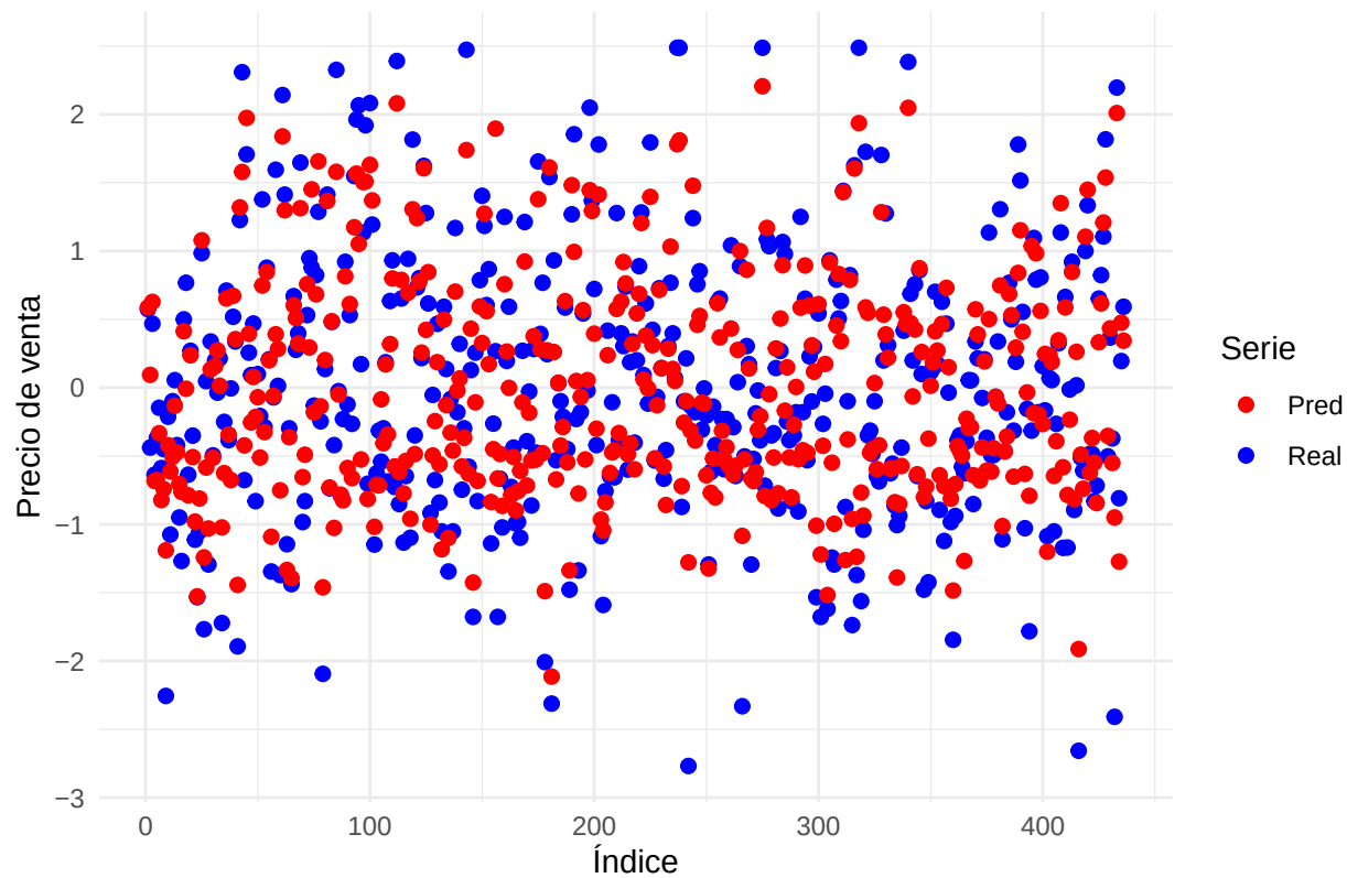
Comparación de valores reales y predichos (Modelo KNN Tunado)
