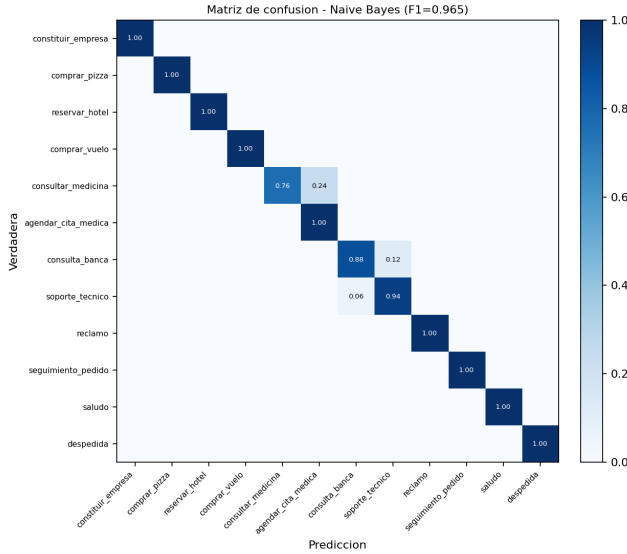
Figura 4. Matriz de confusión del mejor modelo (Naive Bayes), normalizada por clase verdadera. El error se concentra en los pares consultar_medicina/agendar_cita_medica y consulta_banca/soporte_tecnico .
