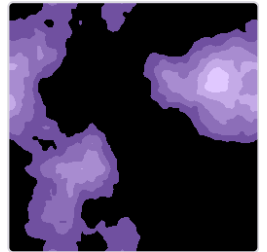
sky_near
