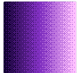
dither
