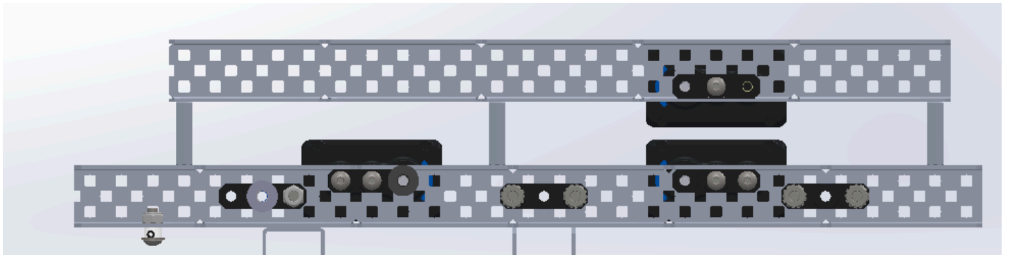
安装机器内边的 25孔窄C，然后安装上置电机 电机与轴承座在同一孔
