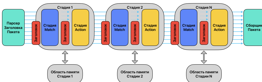
Рис. 1: Общая архитектура конвейера RMT.
