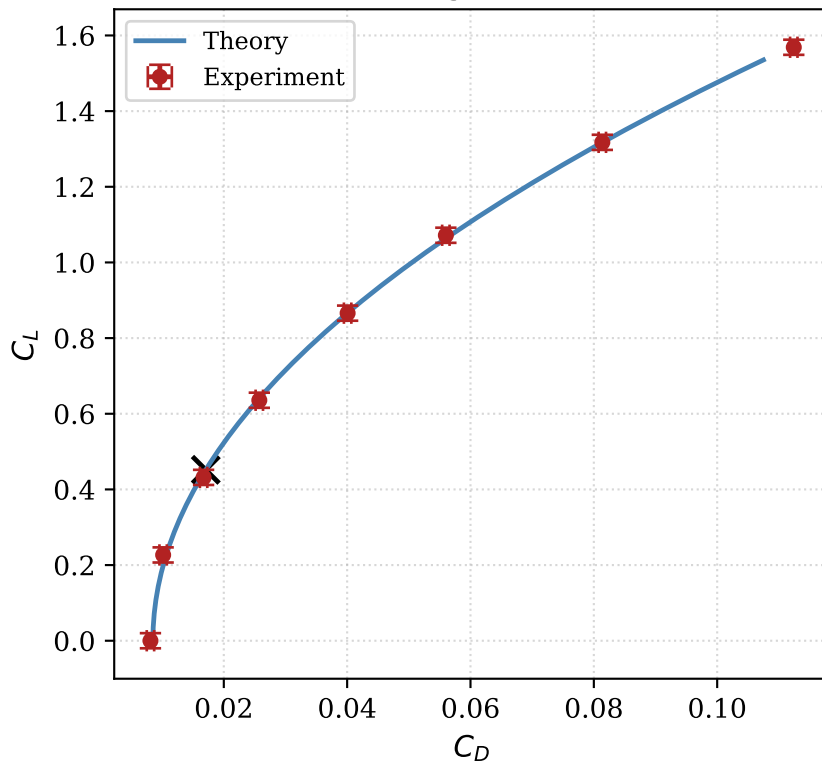
Drag polar
