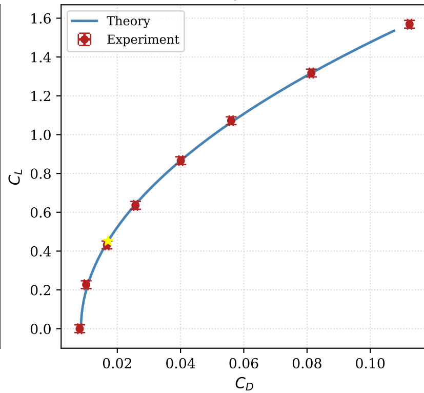
Drag polar
