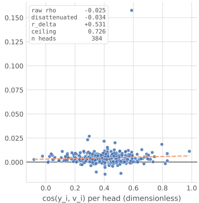
pythia-410m
