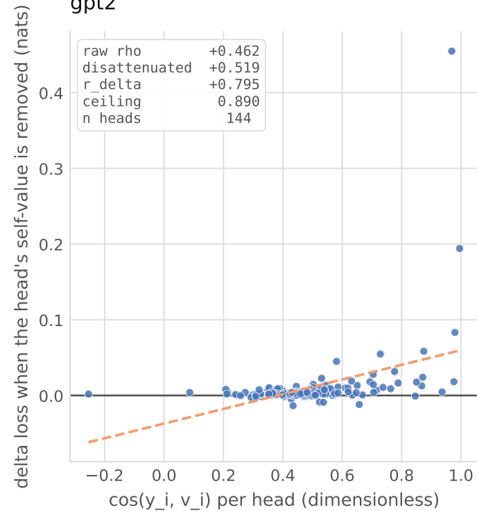
gpt2
