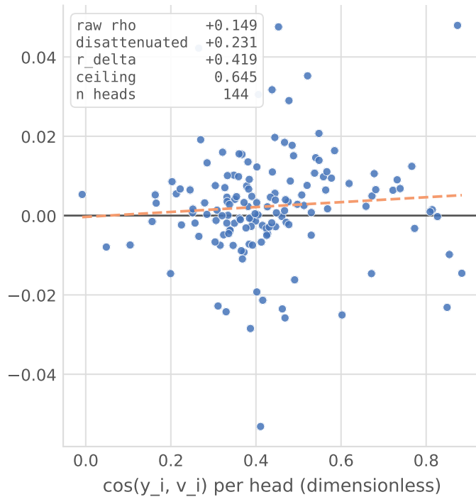
pythia-160m
