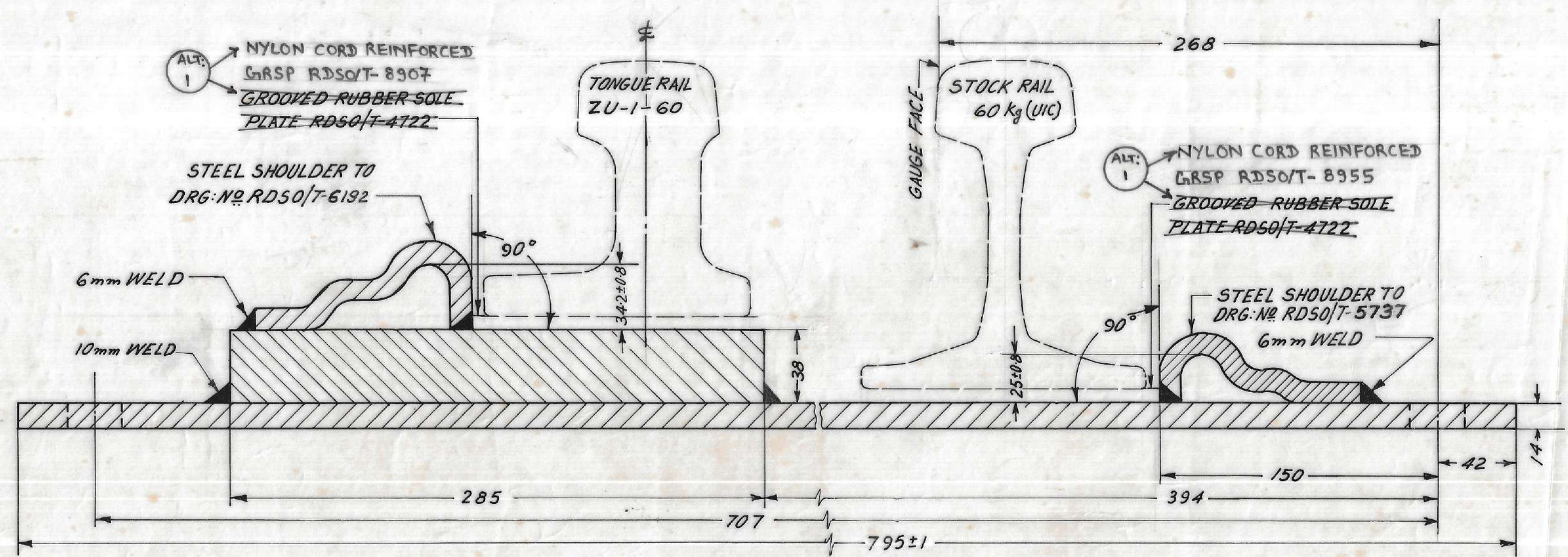
SECTIONAL ELEVATION ON A. B.
