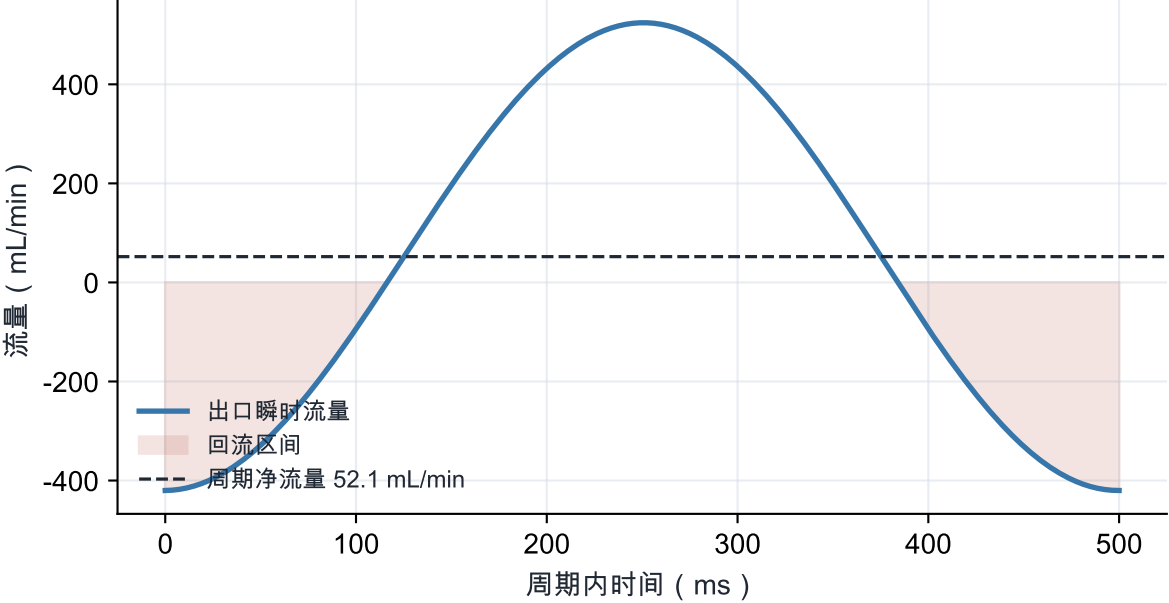
B 2.0 Hz 稳态周期流量
