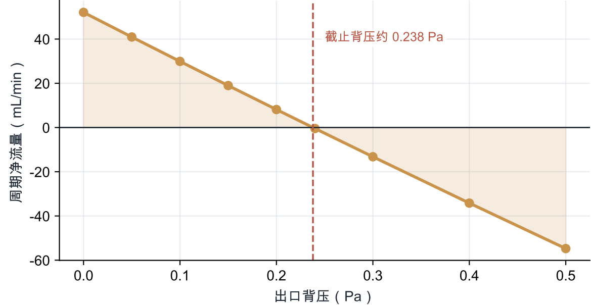
D 2.0 Hz 背压—净流量关系
