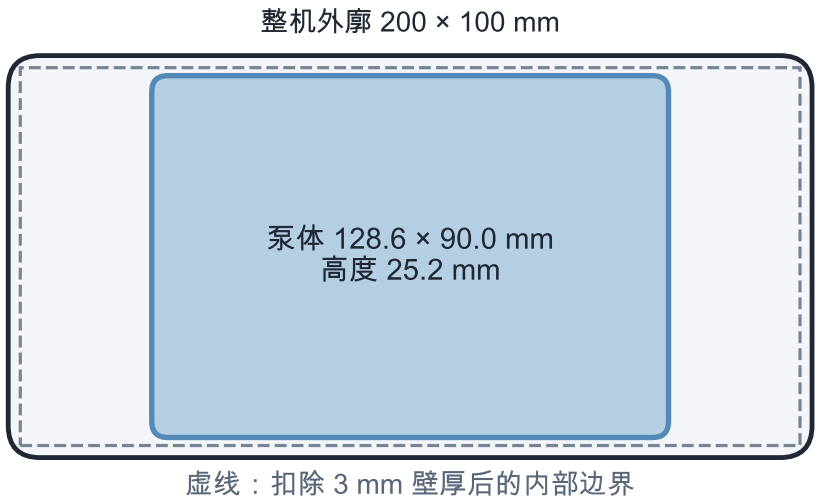
A 装置与缩放泵体包络（俯视）
