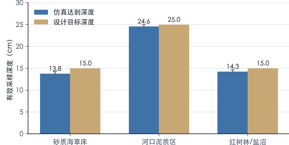
C 典型场景的有效采样深度
