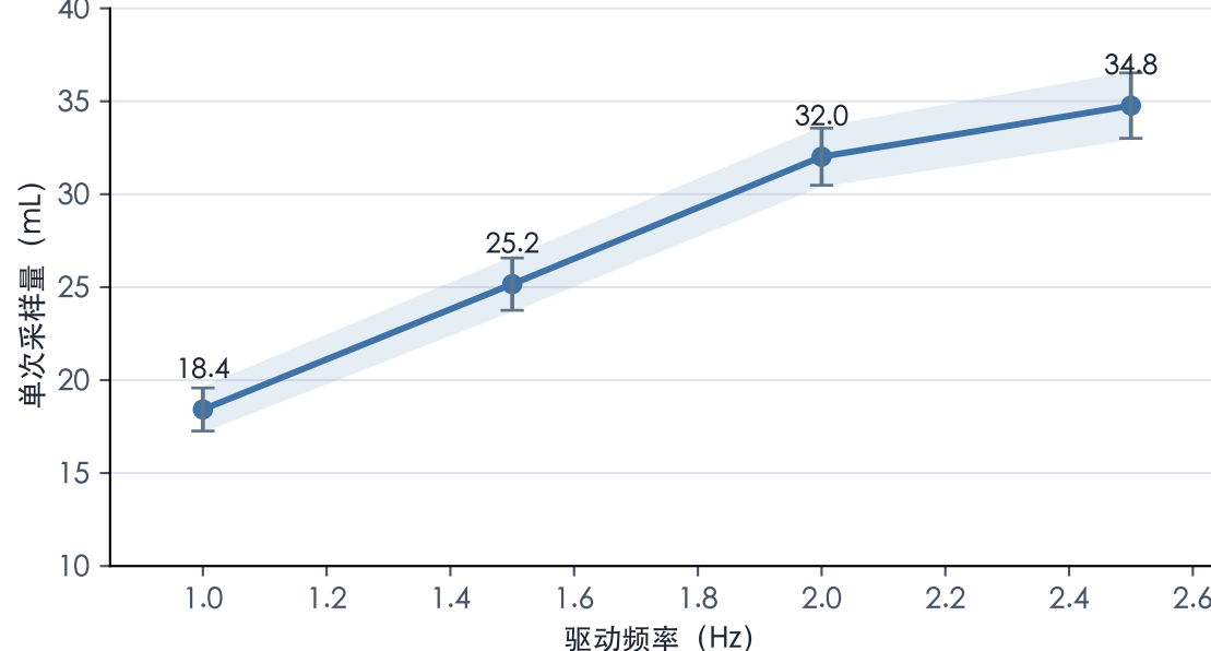
B 驱动频率与单次采样量
