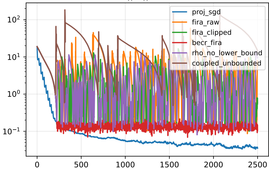
(d) s_t (applied)
