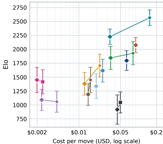
(b) LLMs
