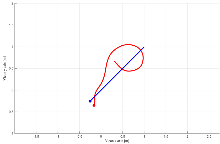
Figura 5: Traiettoria di intercettazione in scenario rettilineo con guida Ibrida.
