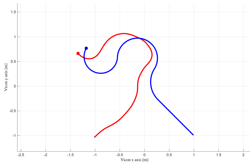
Figura 8: Traiettoria di intercettazione in scenario accelerante con guida PNG.
