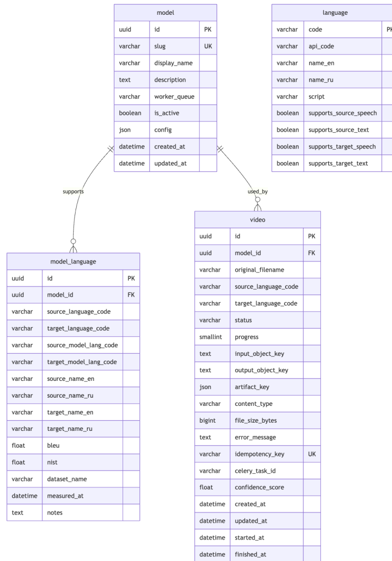
Рис. 5: Схема данных.
