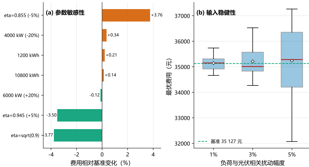
图 11 参数敏感性与输入稳健性
