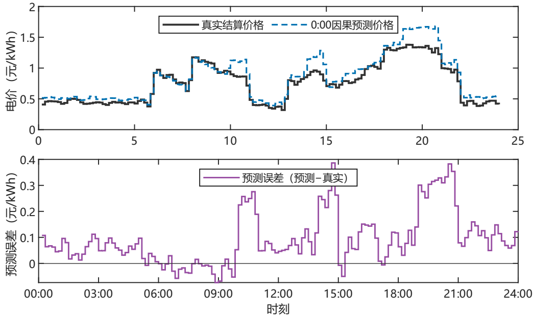
图 9 波动电价下典型日预测价格与真实结算价格对比
