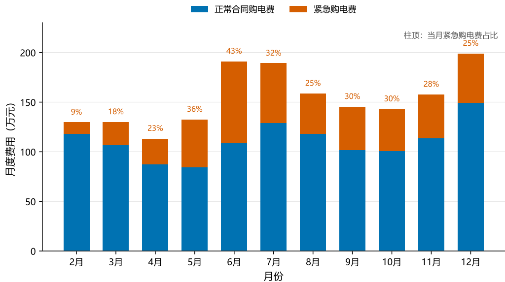
图 4 问题二各月正常合同费用与紧急购电费用构成
