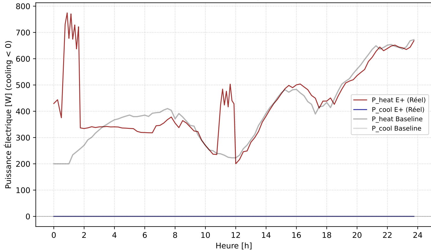
Courbes Puissances Électriques - 2025-03-01
