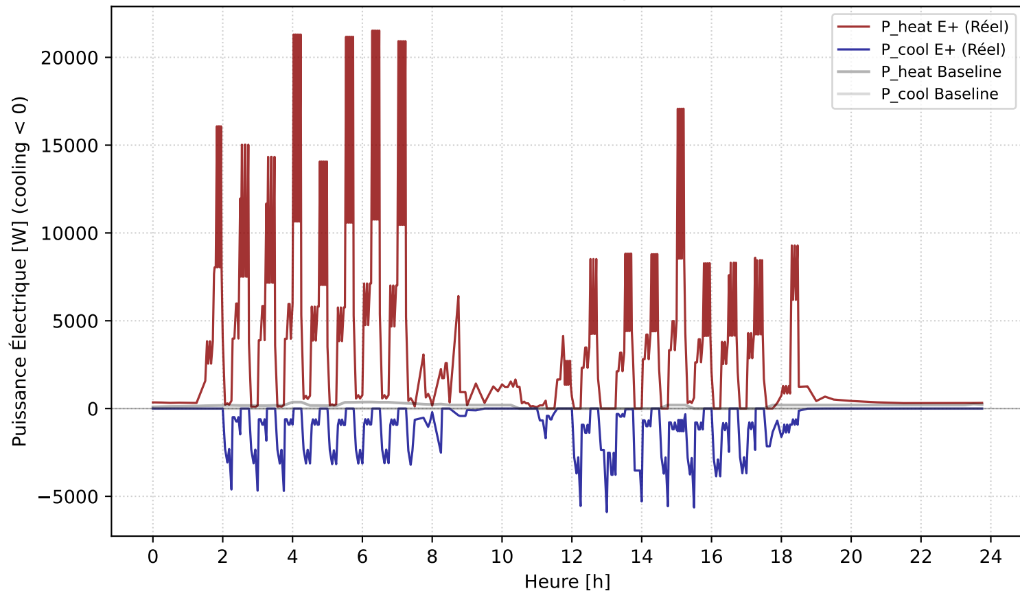
Courbes Puissances Électriques - 2025-10-04
