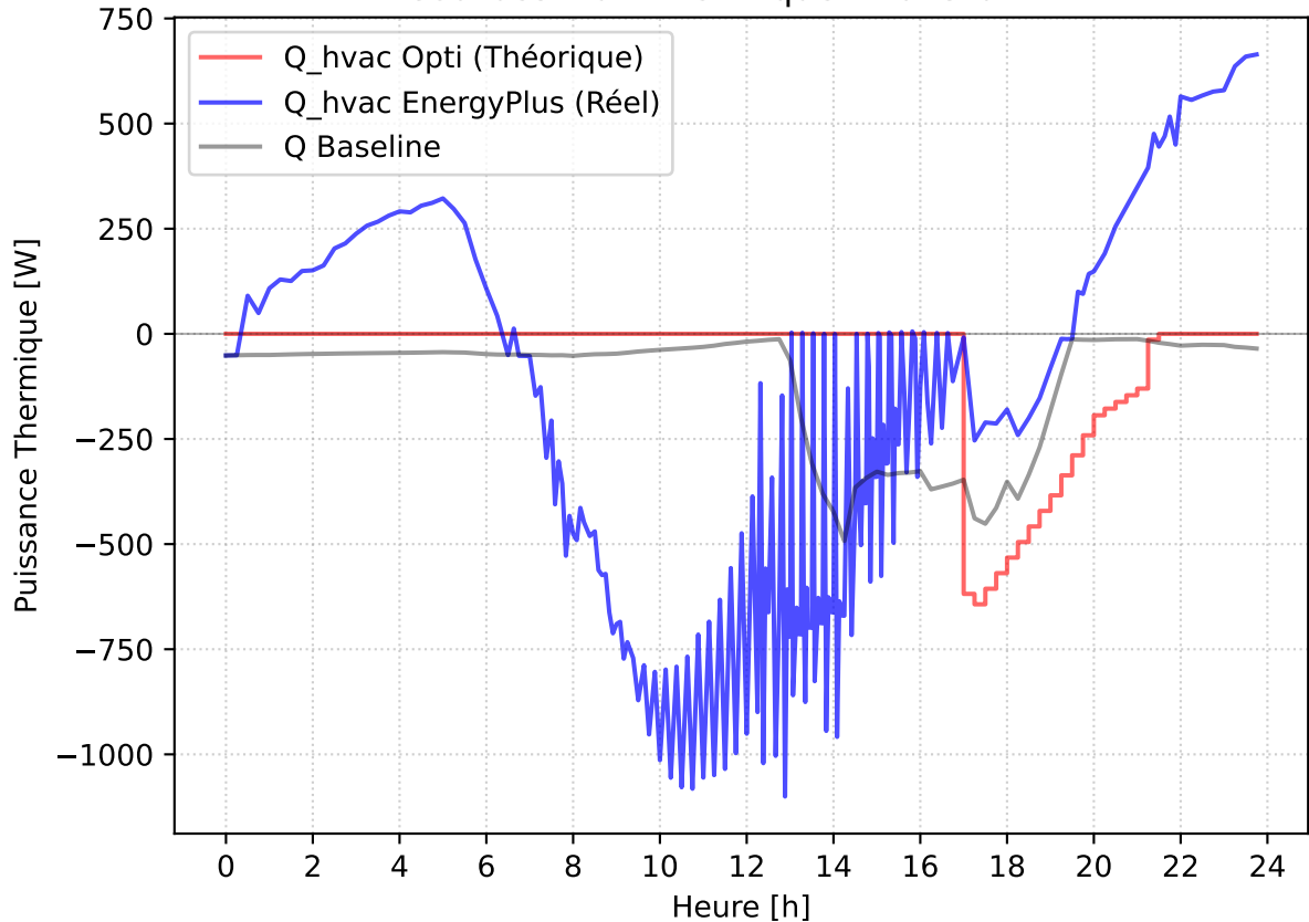
Courbes Flux Thermique - 2025-04-24
