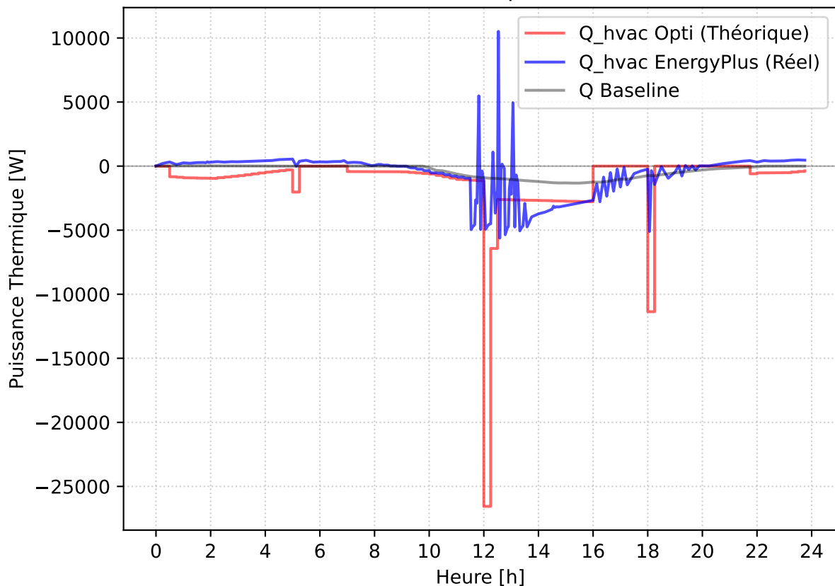
Courbes Flux Thermique - 2025-05-09
