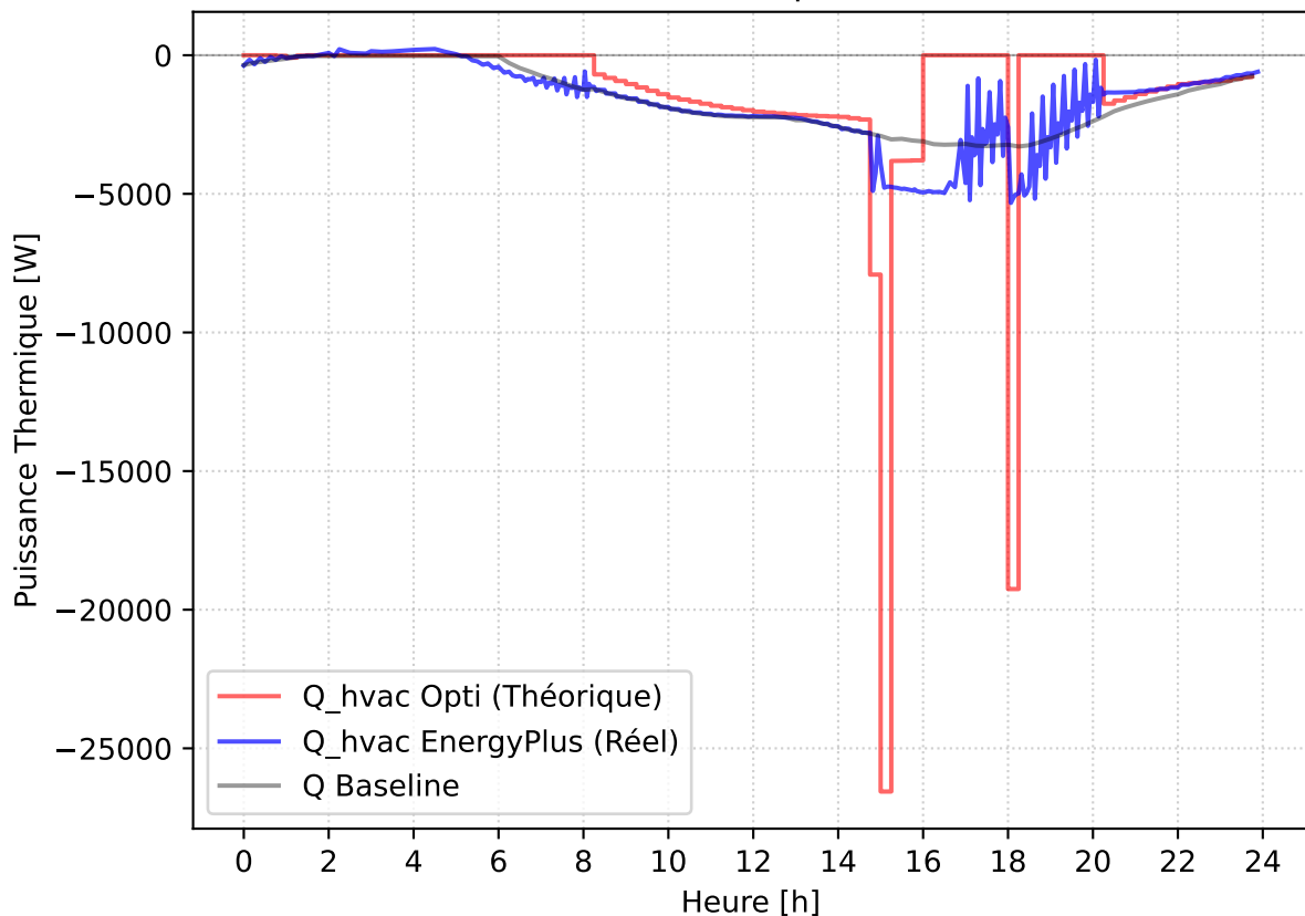
Courbes Flux Thermique - 2025-07-08
