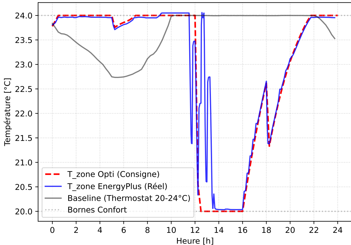
Courbes Températures - 2025-05-09
