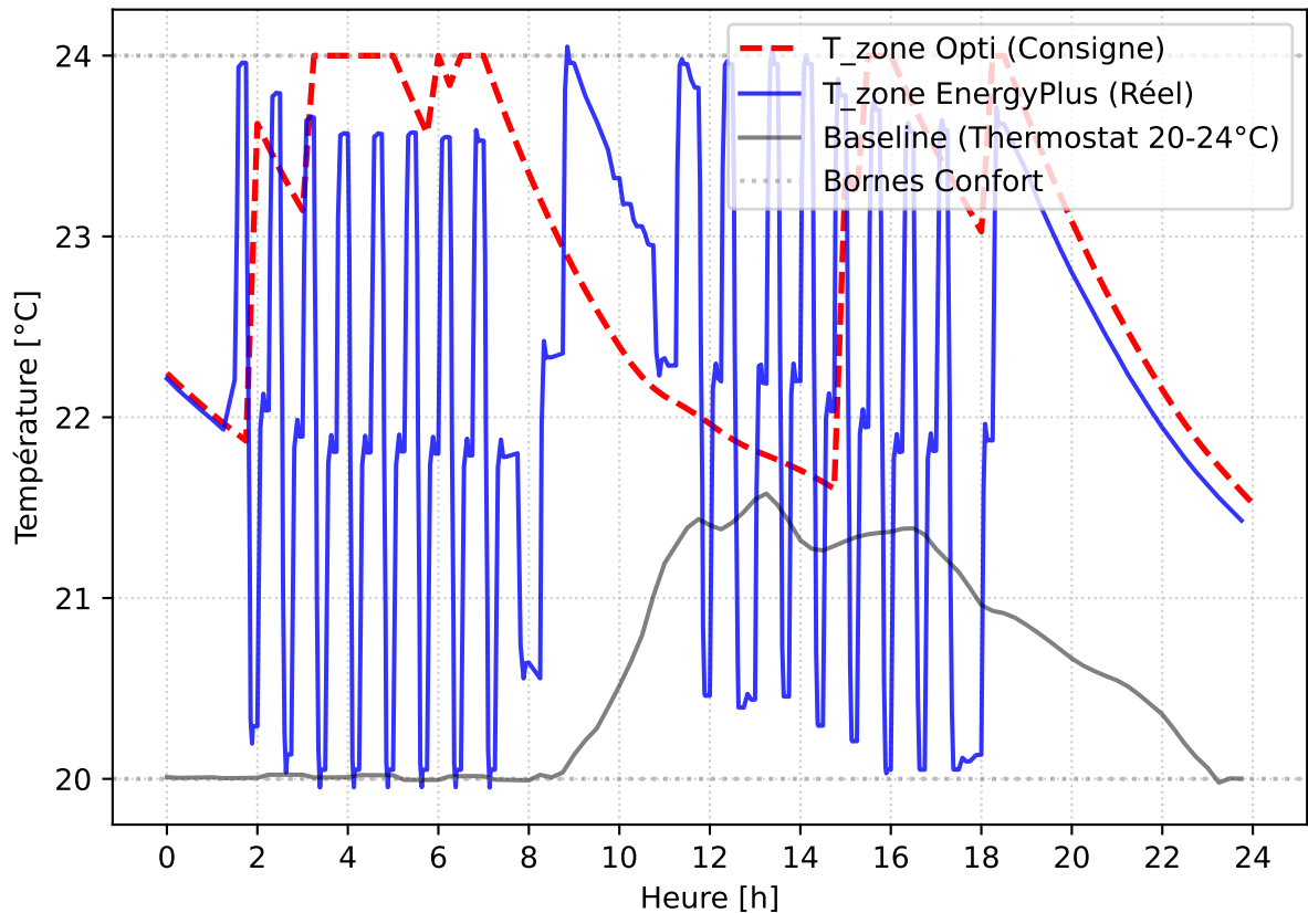
Courbes Températures - 2025-10-04
