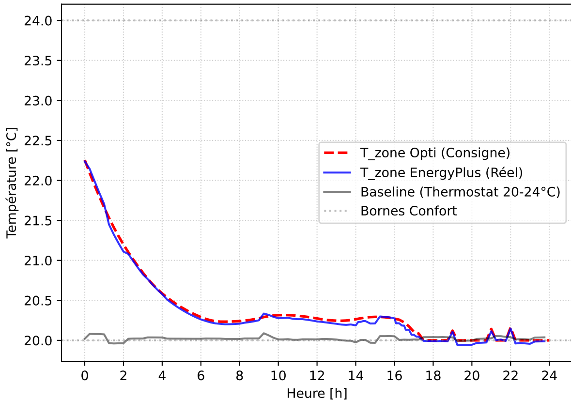
Courbes Températures - 2025-11-22
