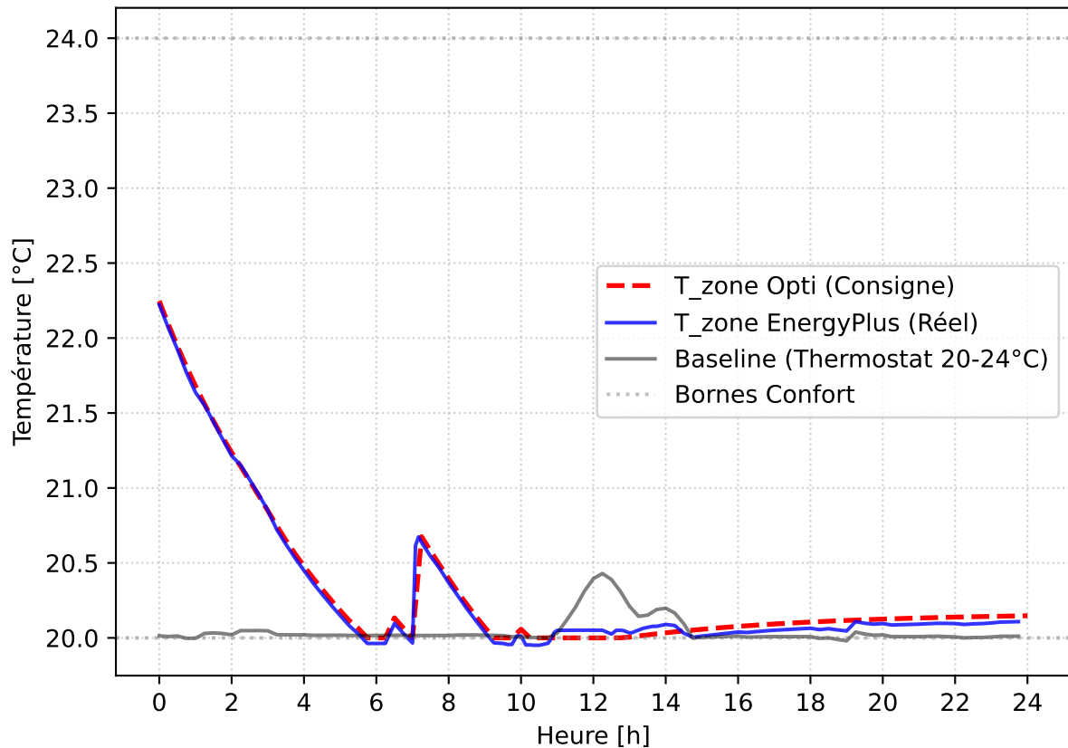
Courbes Températures - 2025-12-24
