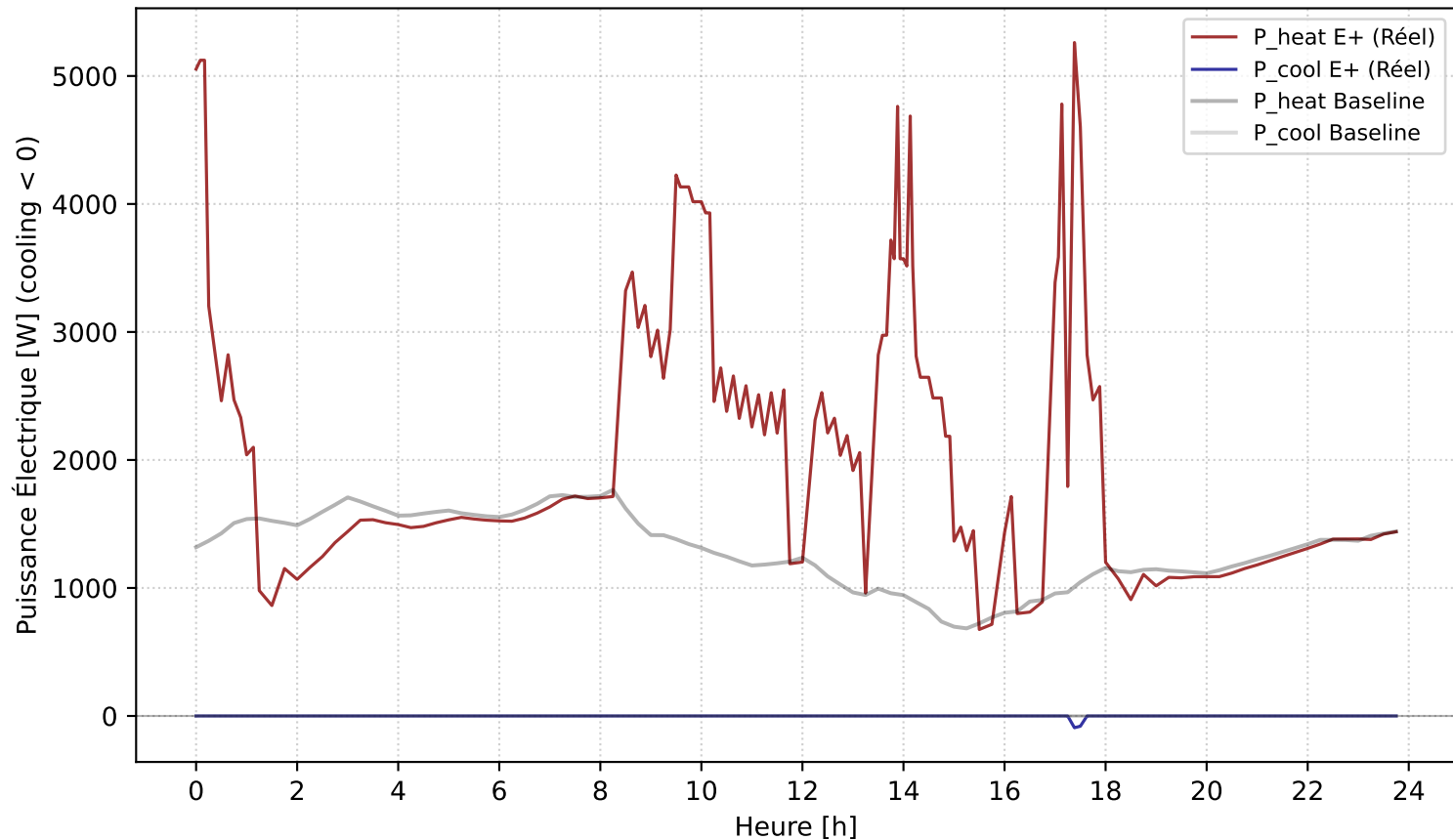
Courbes Puissances Électriques - 2025-02-04
