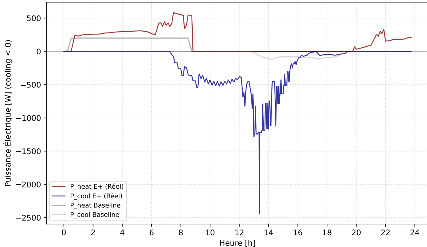
Courbes Puissances Électriques - 2025-04-24
