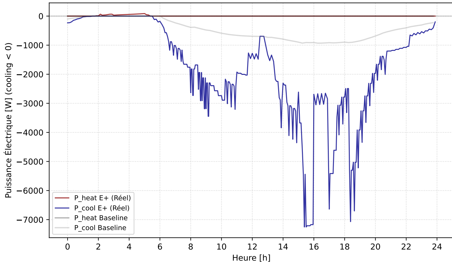
Courbes Puissances Électriques - 2025-07-08
