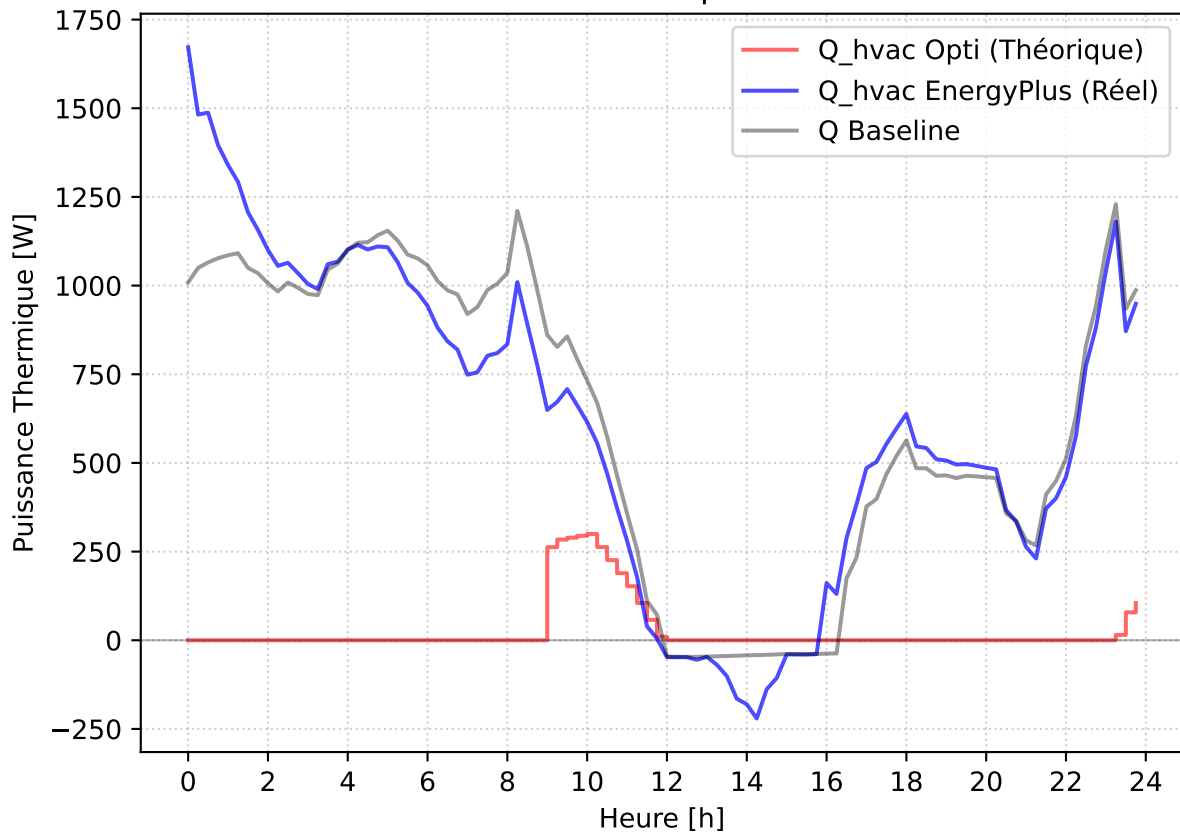
Courbes Flux Thermique - 2025-01-21
