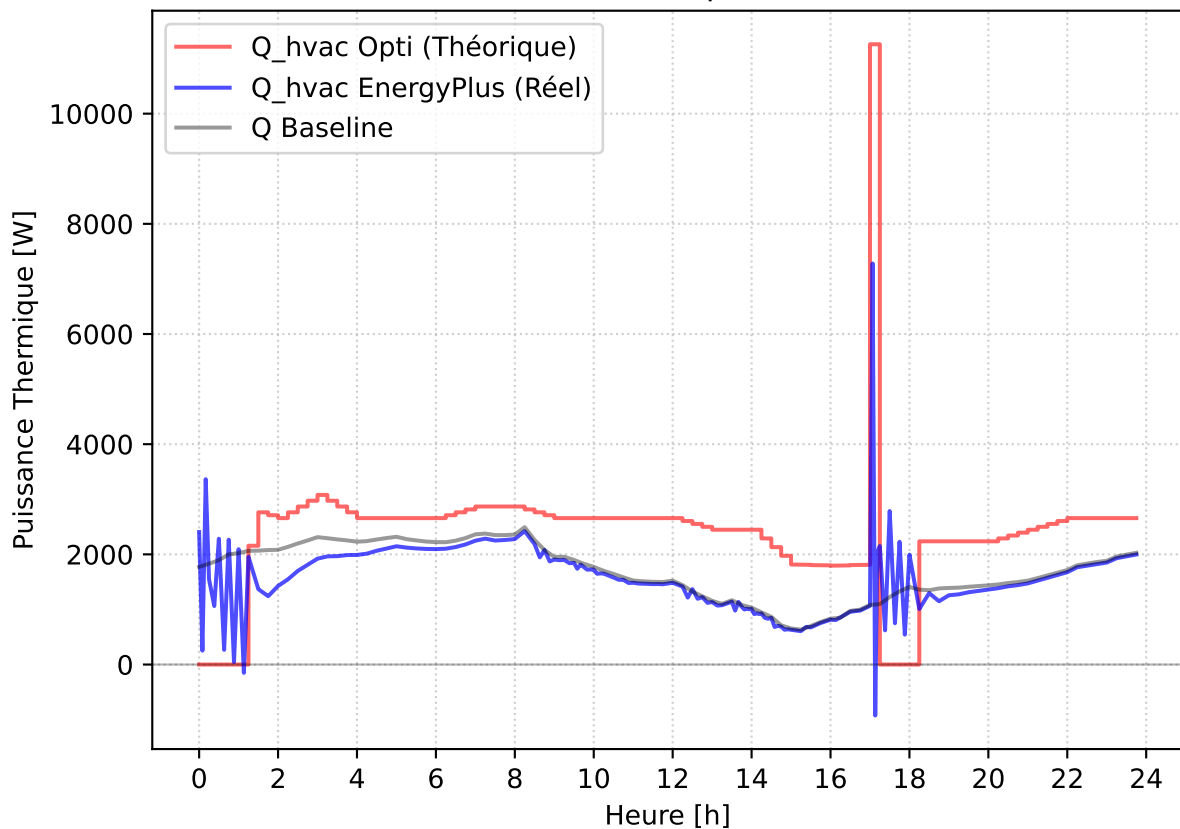
Courbes Flux Thermique - 2025-02-04
