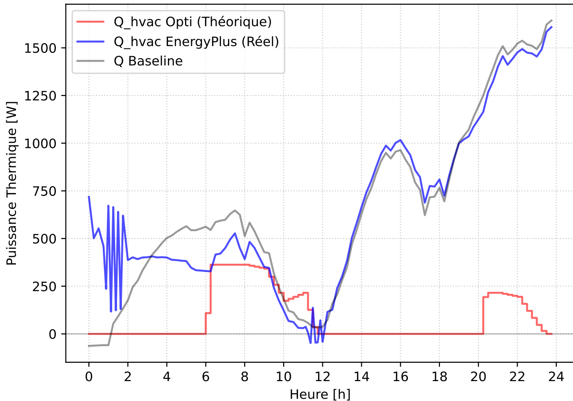
Courbes Flux Thermique - 2025-03-01
