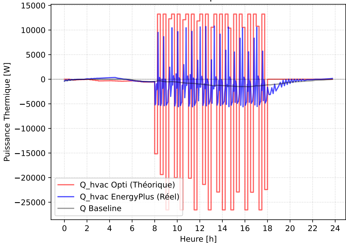
Courbes Flux Thermique - 2025-06-08
