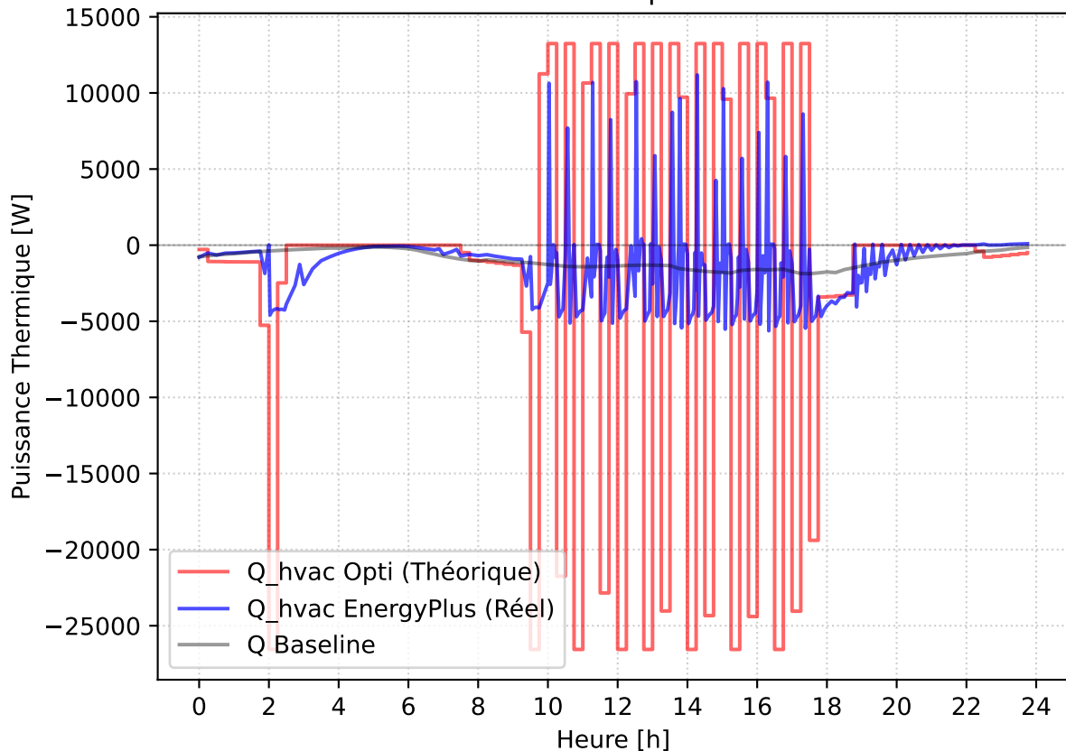
Courbes Flux Thermique - 2025-08-05
